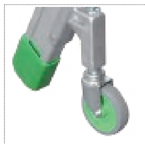
Ruote anteriori Ø 80 mm piroettanti, autofrenanti
